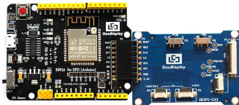
图 3 转接板与主板连接方式
