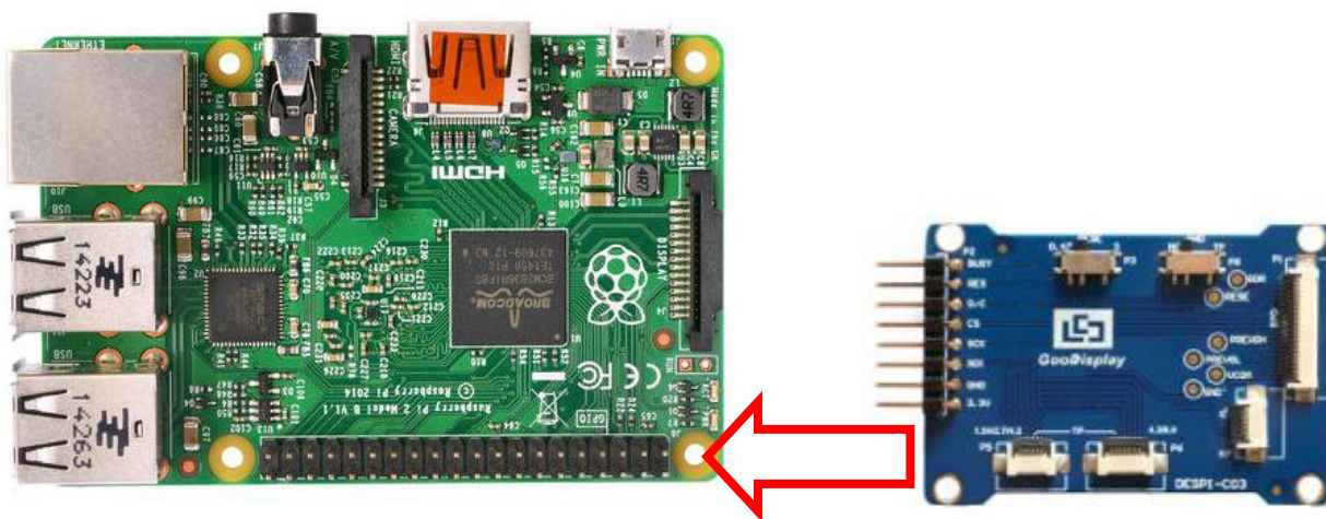
图 7 转接板与树莓派连接方式
