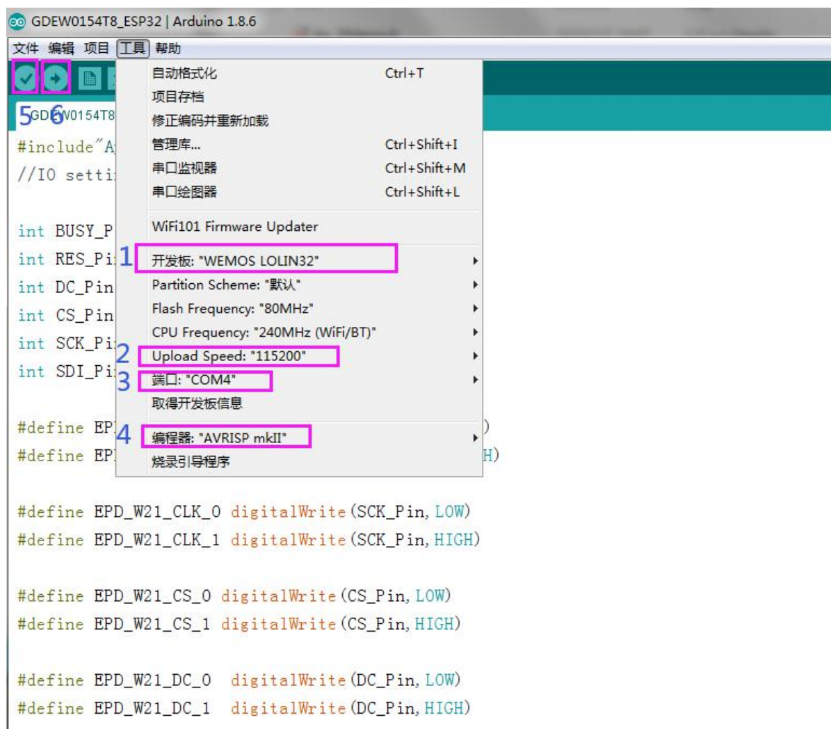
图 10 程序下载操作步骤
